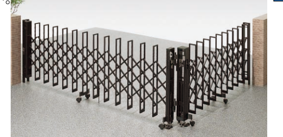
MB型 両開き角地納まり
