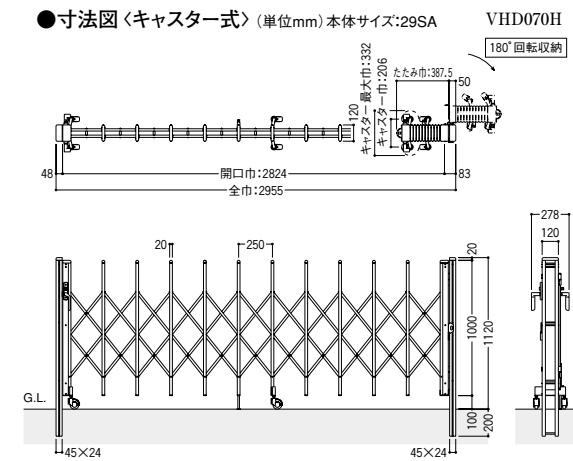
キャスター式 両開き角地タイプ 写真はセレビューMB型です。 [CBブラック]
