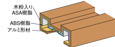
図は木樹脂フェンス用柱端部材です。
