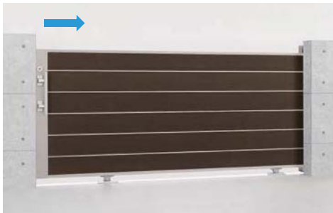
片引きタイプ シャイングレー+柿渋 手動タイプ 30-12型 全幅=3,000mm 高さ=1,200mm
